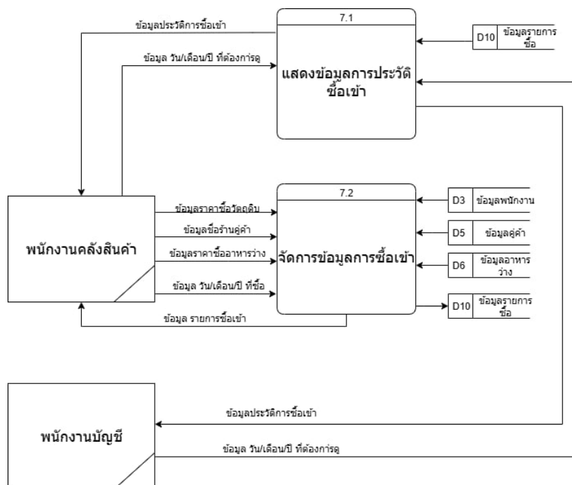
ภาพที่ 3.8 DFD_level1_7.0
