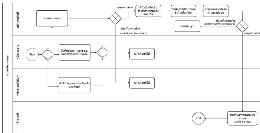
ภาพที่ 3.4 แสดงแผนผังการทำงานในระบบงานใหม่
