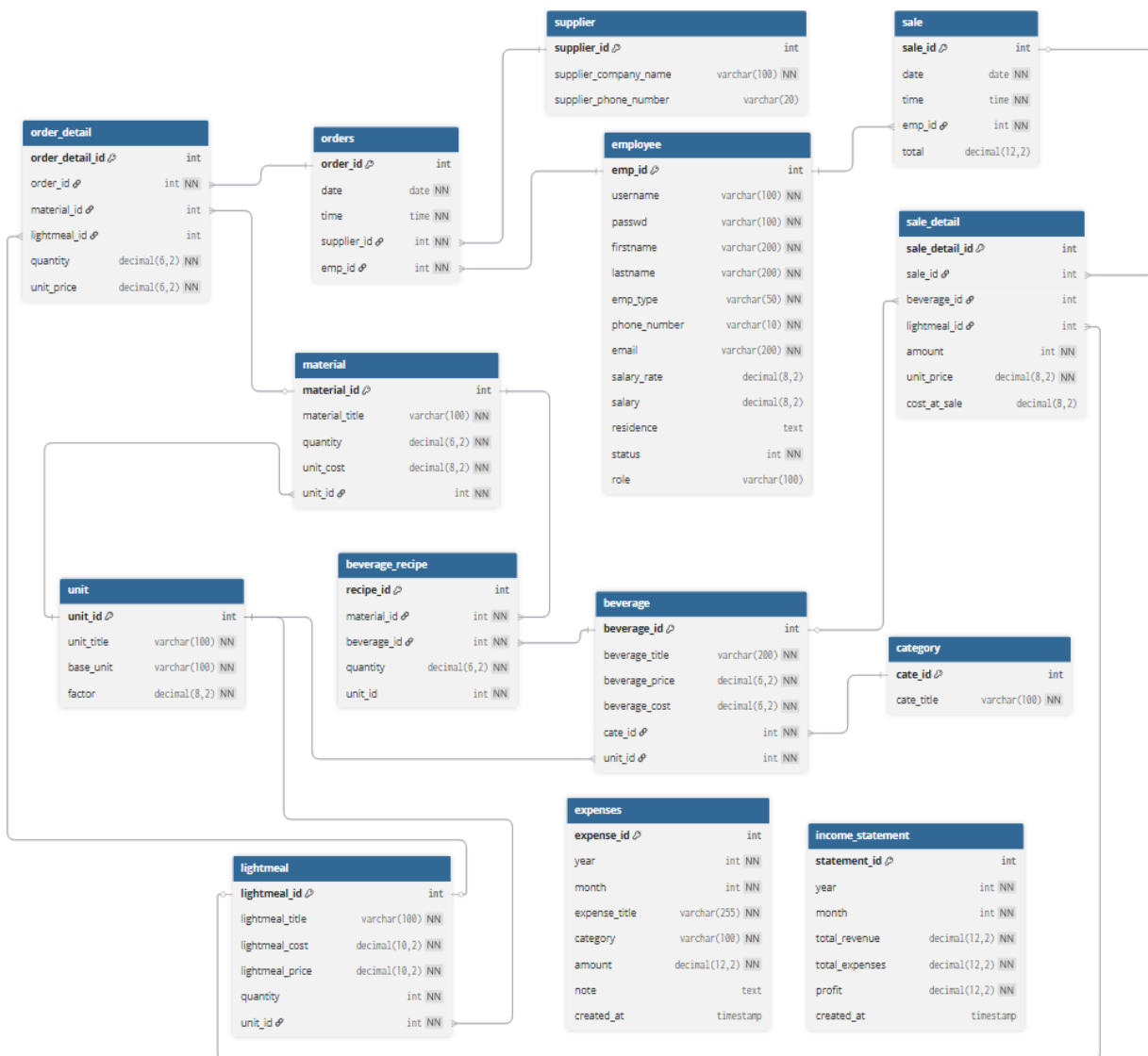
ภาพที่ 3.13 ER_Diagram
