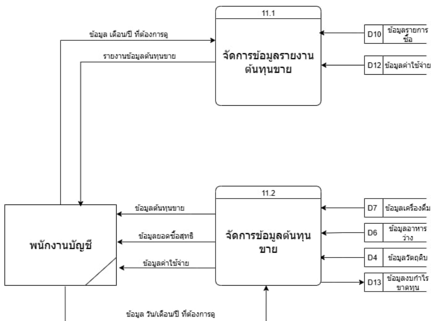
ภาพที่ 3.11 DFD_level1_11.0
