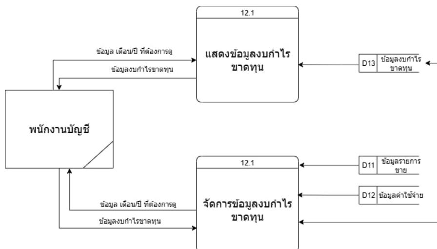
ภาพที่ 3.12 DFD_level1_12.0
