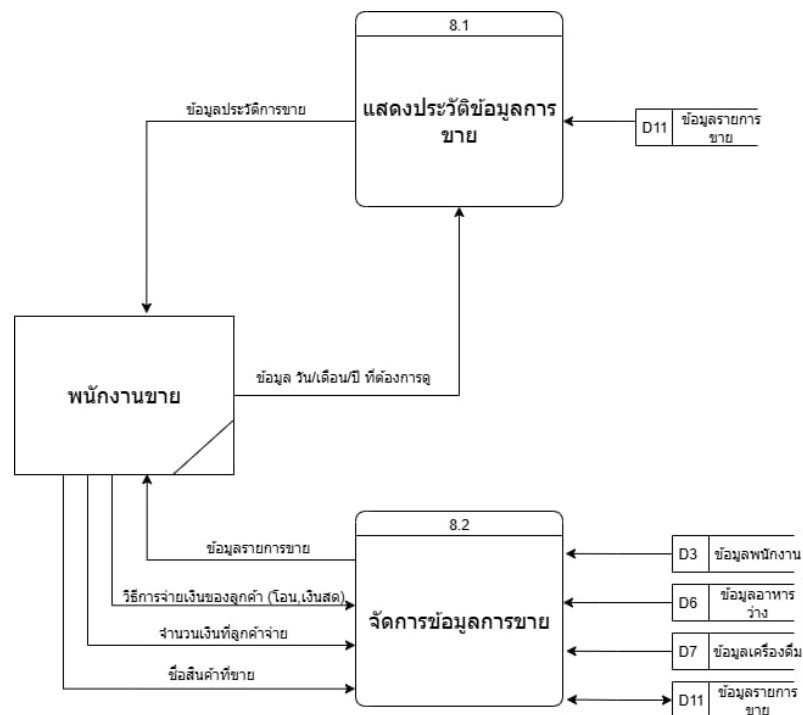
ภาพที่ 3.9 DFD_level1_8.0
